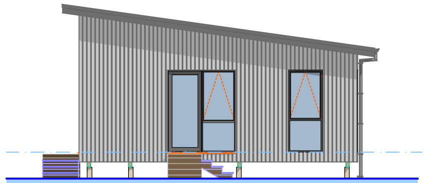
D Elevation 1:100
