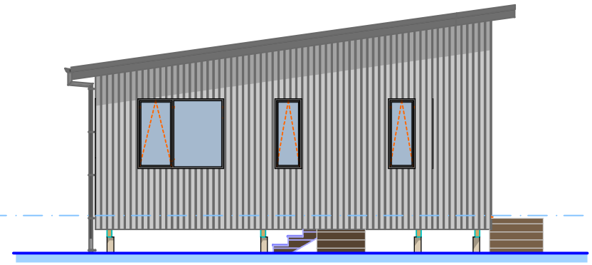
B Elevation 1:100
