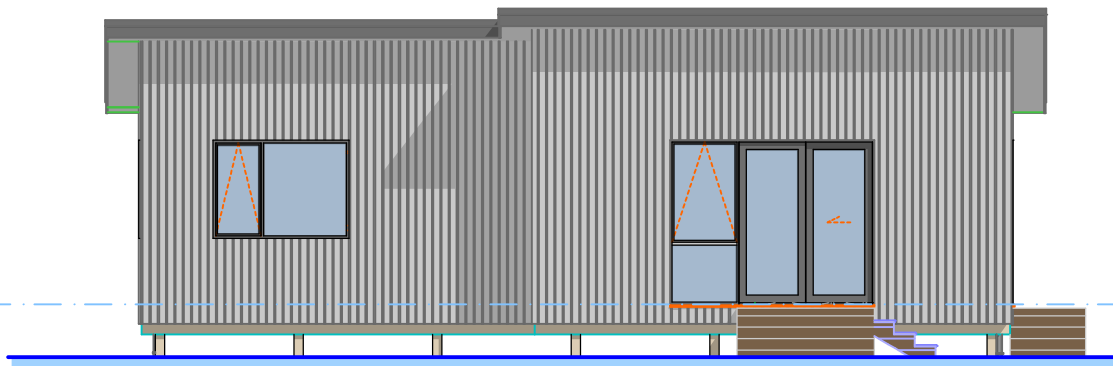
C Elevation 1:100
