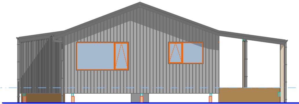
C Elevation 1:100
