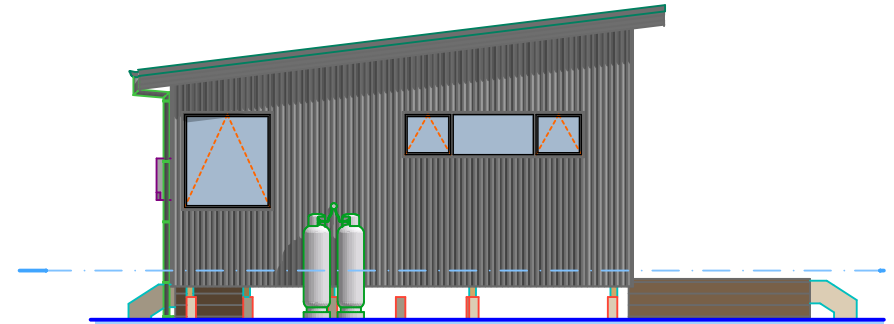
B Elevation 1:100
